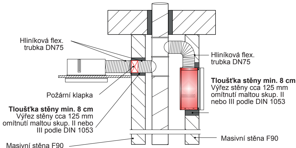
Obr. 21: tloušťky stěn nejméně 80 mm
