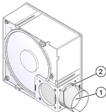
Obr. 29: Zpětná klapka - výstup bočně doleva
