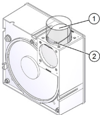
Obr. 28: Zpětná klapka - výstup bočně vzhůru
